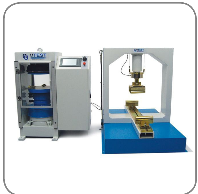
Presse de compression avec bâti de flexion
